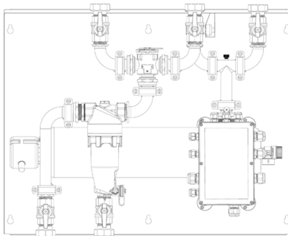
Abbildung 17. Montagevorlage
