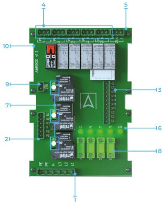
Abbildung 5. Beschreibungen auf der Leiterplatte
