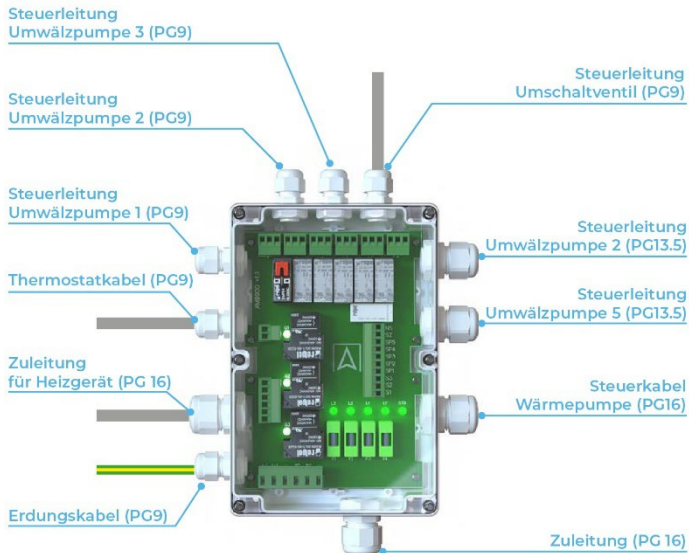
Abbildung 7. Markierungen auf Kabelverschraubungen
