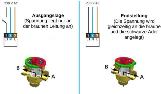
Abbildung 12. Position des Dreiwegeventils
