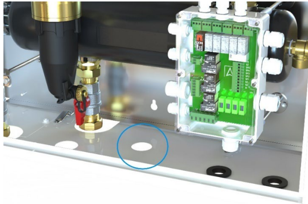
Abbildung 20. Auslassöffnung des Sicherheitsventils
