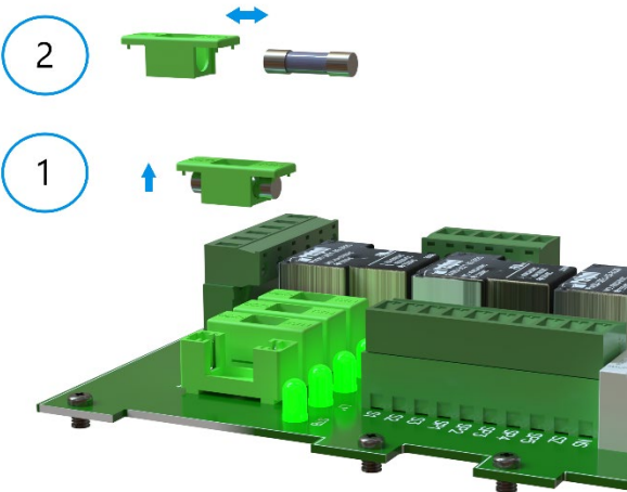
Abbildung 29. Austausch einer Sicherung
