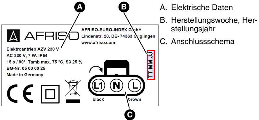
Abbildung 1: Beispiel Typenschild
