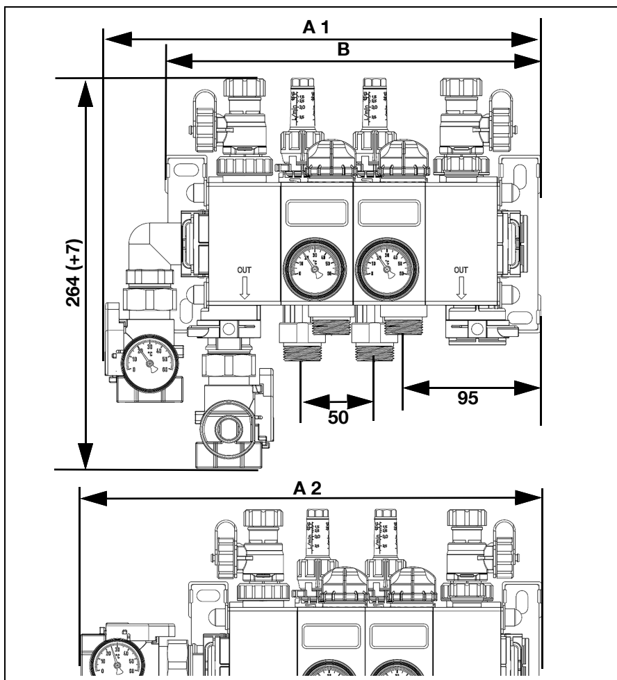
Ilustracja 1: Wymiary [mm]
