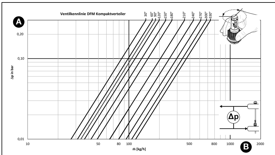
Ilustracja 4: Krzywe strat ciśnienia w zależności od przepływu i stopnia otwarcia rotametu zamontowanego na rozdzielaczu. Uwzględniono stratę ciśnienia na zaworze powrotnym
