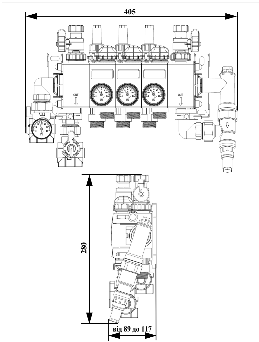
Рисунок 3: Розміри [мм]
