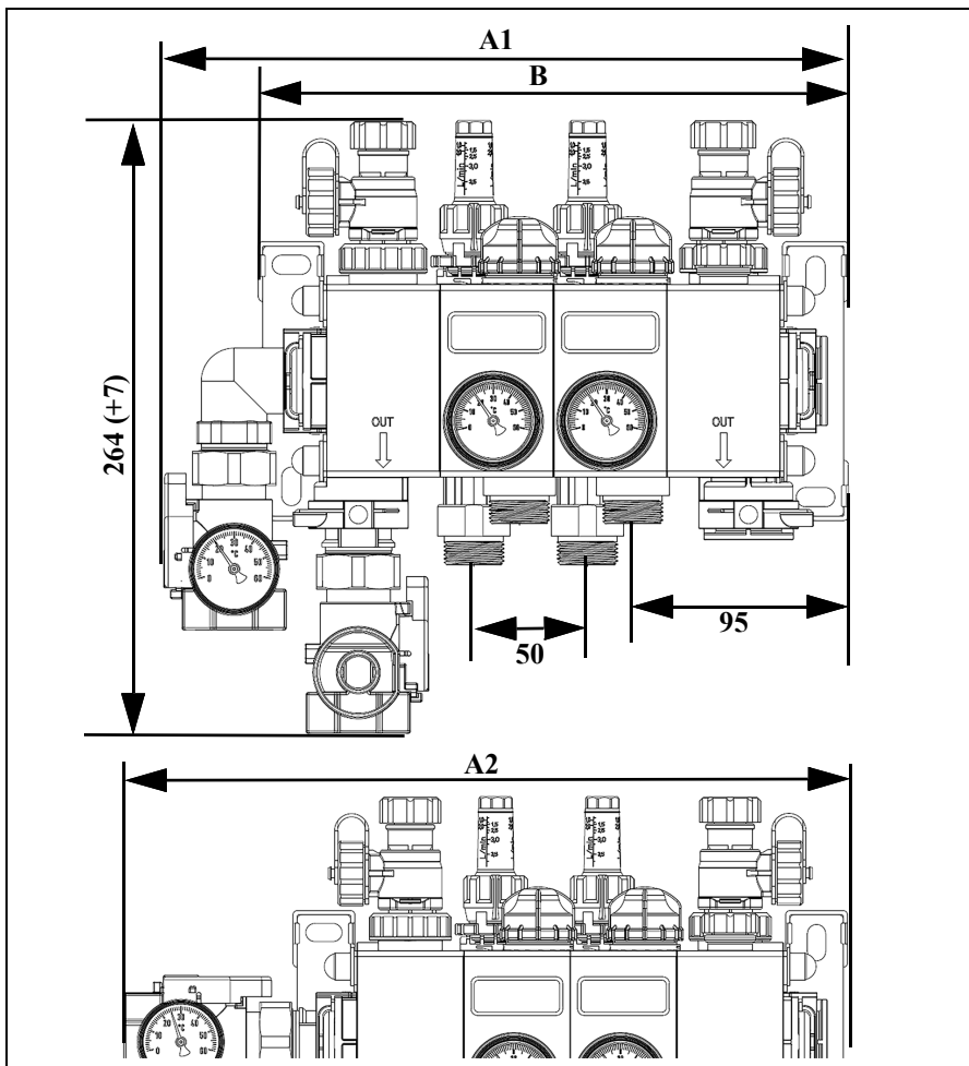
Рисунок 1: Розміри [мм]
