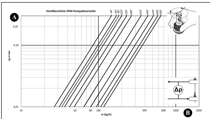
Рисунок 4: Криві зниження тиску залежно від витрати і ступеня відкриття ротаметра, встановленого на колекторі. Зниження тиску на зворотному клапані враховано
