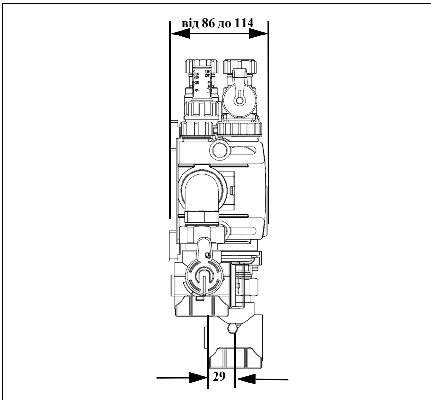
Рисунок 2: Розміри [мм]
