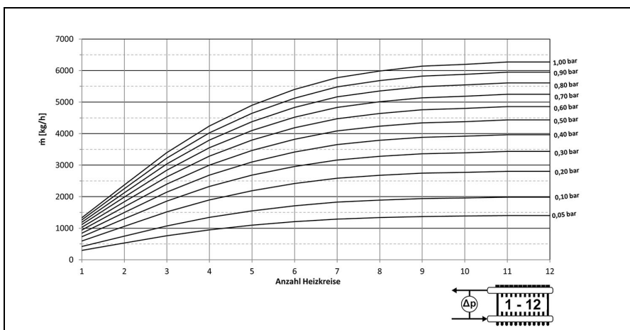
Рисунок 5: Діаграма загального зниження тиску в колекторах із ротаметром
