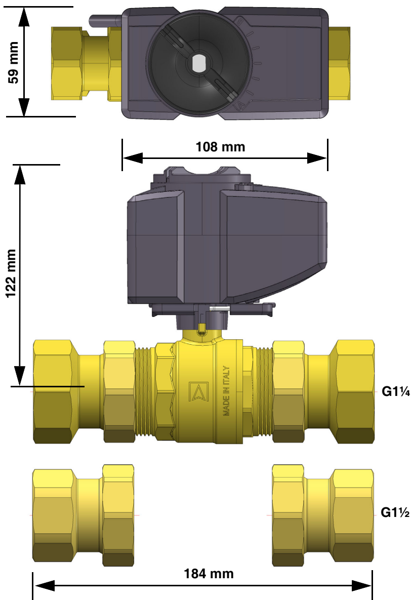
Abbildung 4: Abmessungen Absperrkugelhahn G1½ mit Verschraubungen G1¼ und G1½
