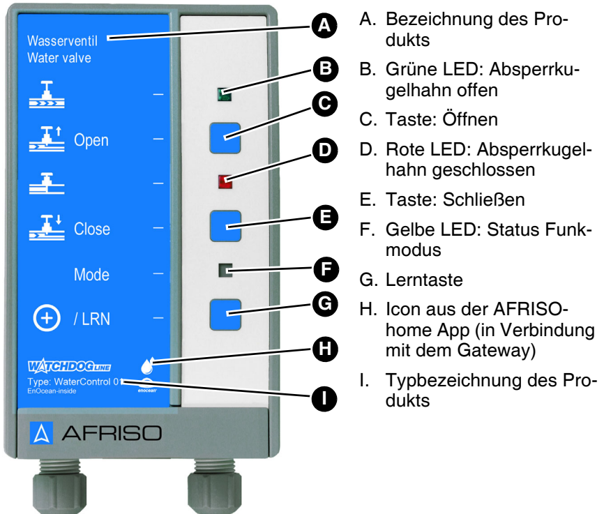
Abbildung 1: Signalteil
