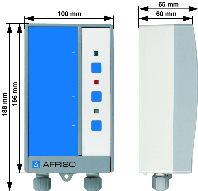
Abbildung 2: Abmessungen Signalteil
