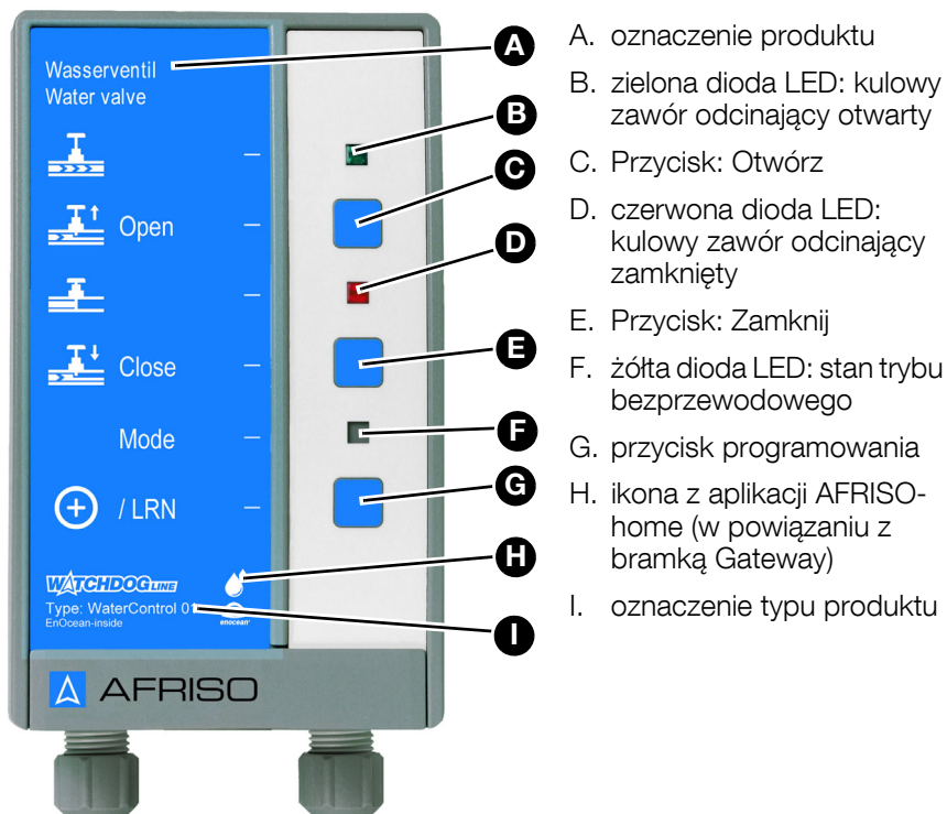
Ilustracja 1: Sygnalizator
