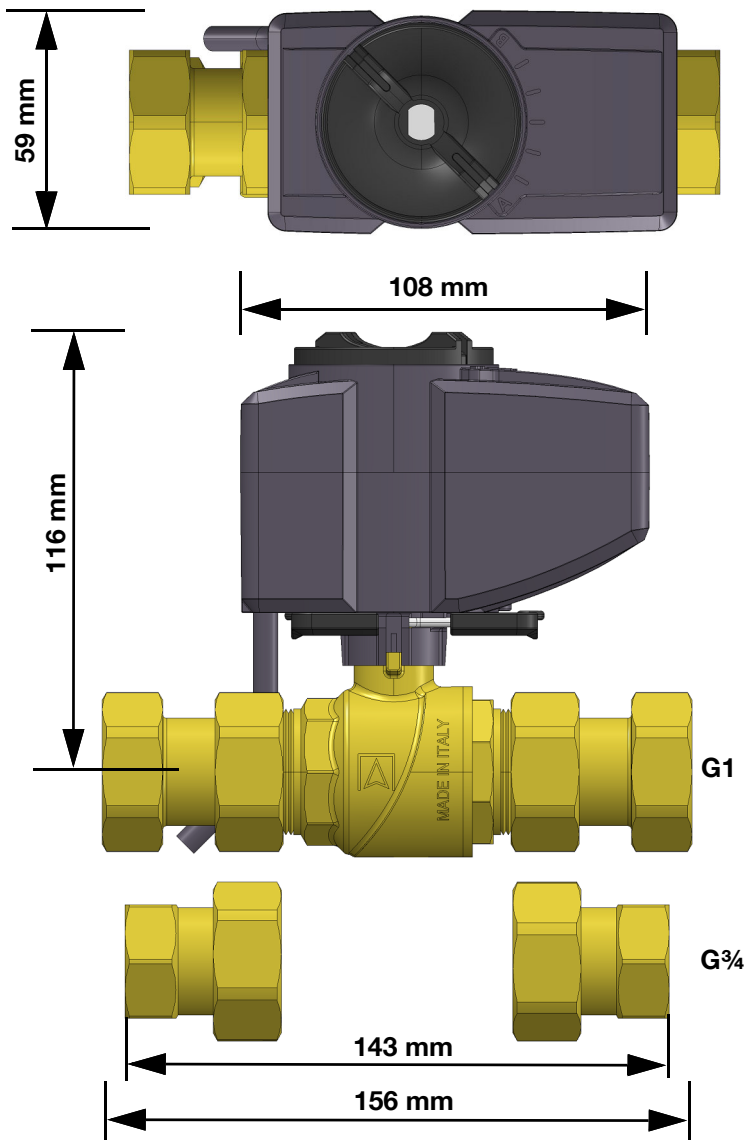
Ilustracja 3: Wymiary kulowego zaworu odcinającego G1 ze śrubunkami G \frac{3}{4} i G1
