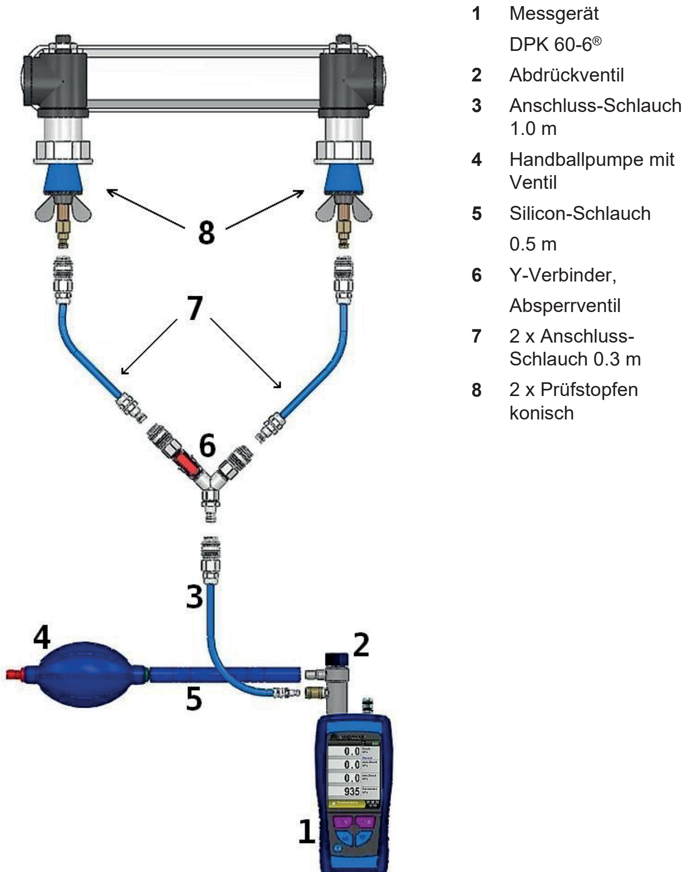
Bild 1: Anschlussschema vom DPK 60-6 (Option)
