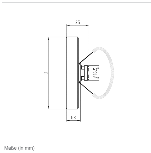
Maße (mm)
