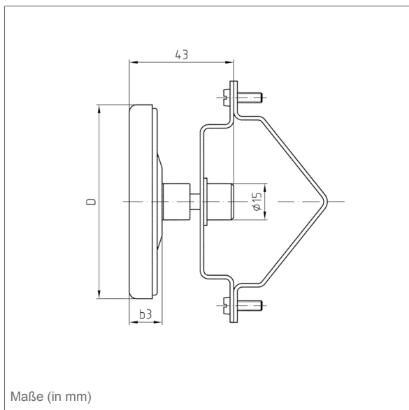
Maße (mm)
