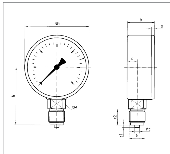
NG 80 – Anschluss radial
