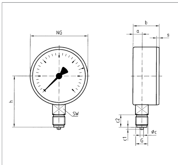
NG 40/50/63 – Anschluss radial
