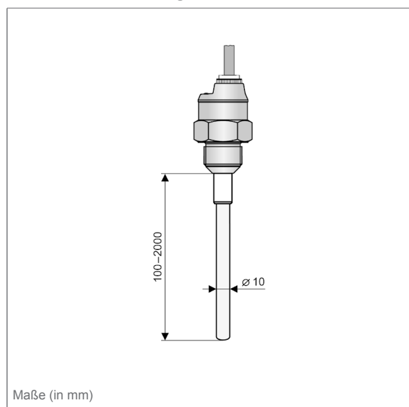
CapFox® EFT 20 MS - 21 mit starrer Monosonde mit FEP-Isolierung – CapFox® EFT 20 MS - 22 mit starrer Monosonde mit PFA-Isolierung
