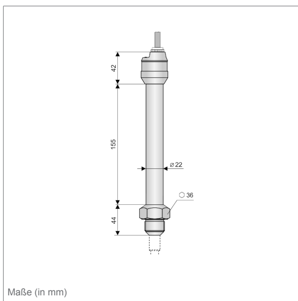
CapFox® EFT 20 Hochtemperatursausführung
