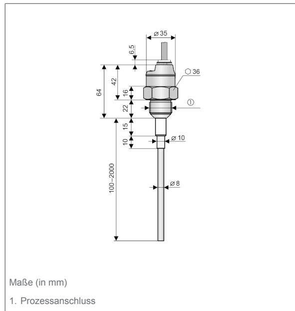
CapFox® EFT 20 MS - 20 mit starrer Monosonde
