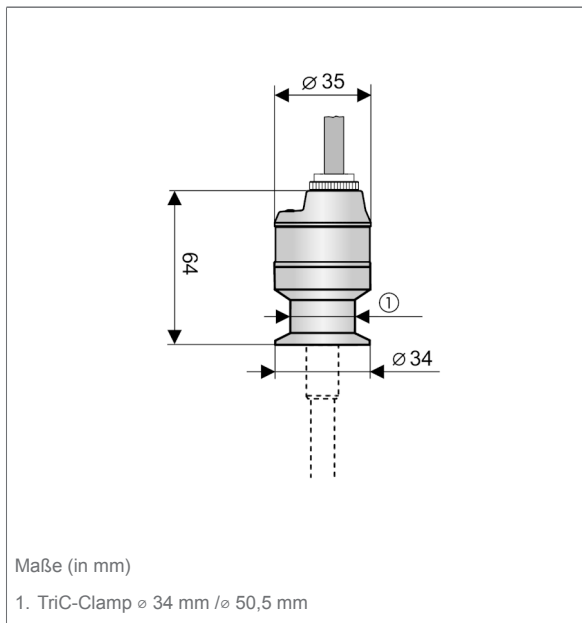
CapFox® EFT 20 Prozessanschluss Tri-Clamp DIN 32676
