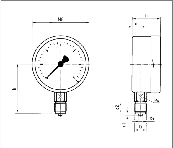
Maße (mm)
