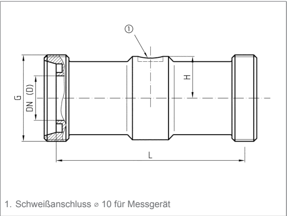
Typ RD 50 - DIN 11851/DIN 11887
