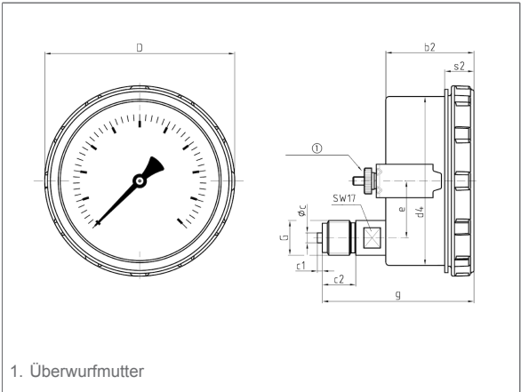
Maße (mm)
