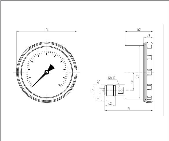
Anschluss axial exzentrisch
