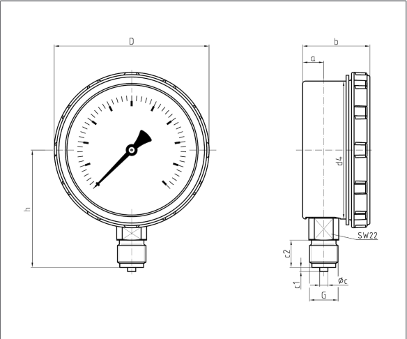
Anschluss radial
