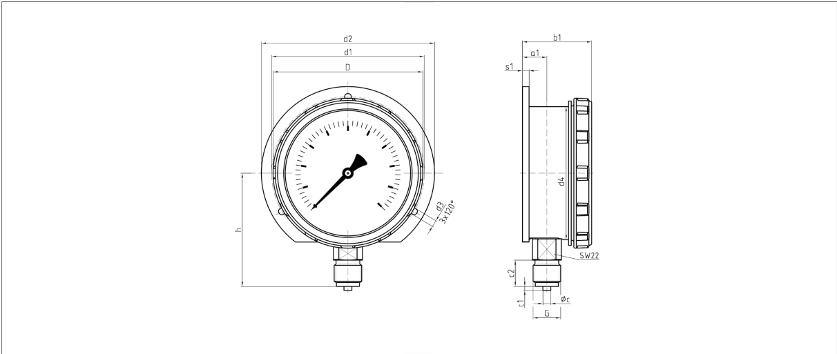
Maße (mm)
