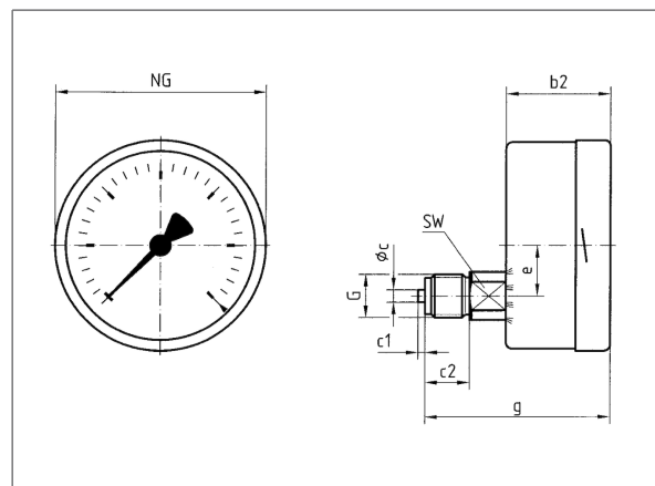
Anschluss axial exzentrisch
