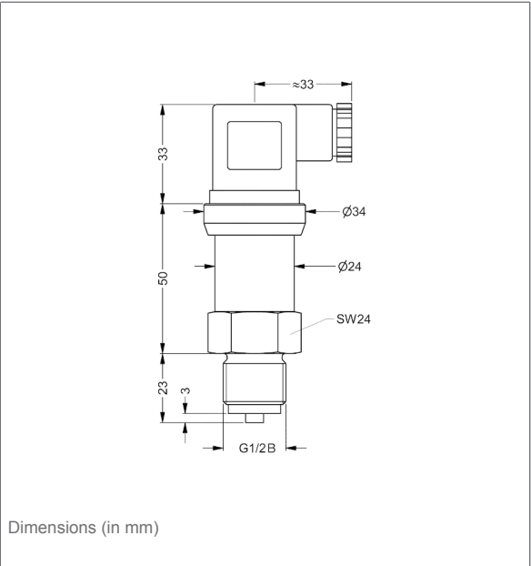
DMU 01 - connection G½B EN 837
