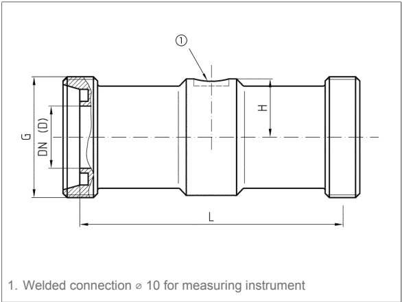
Type RD 50 - DIN 11851/DIN 11887
